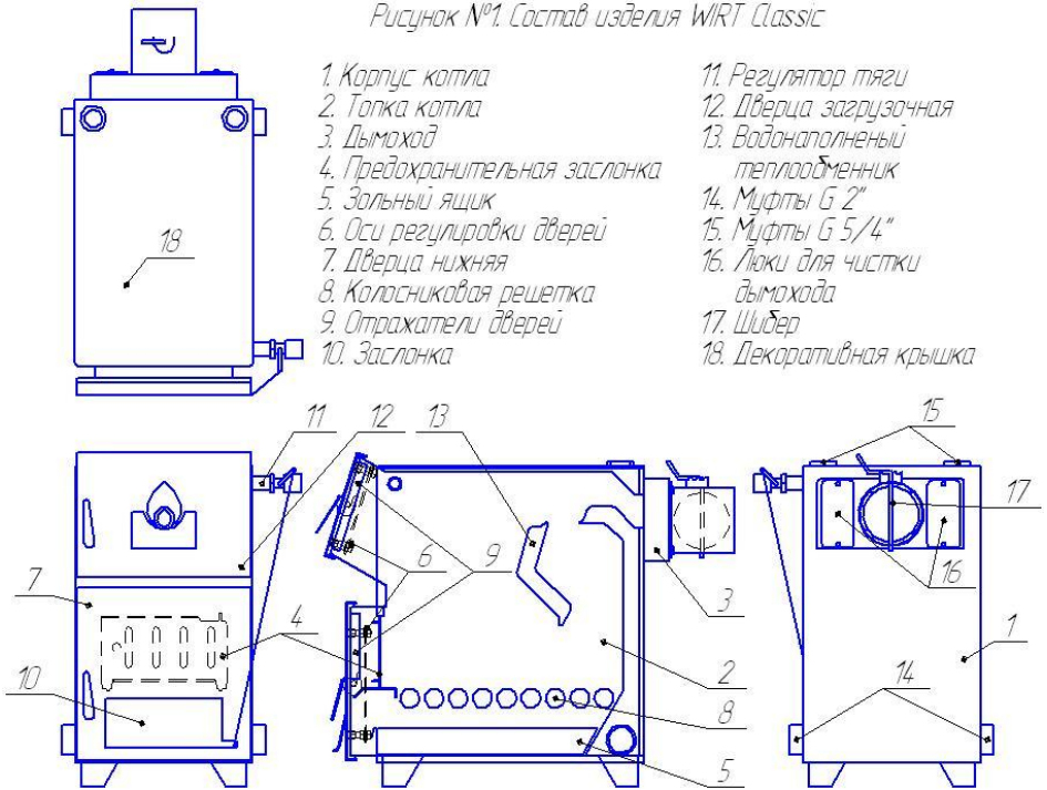
Рисунок №1. Состав изделия WIRT Classic
